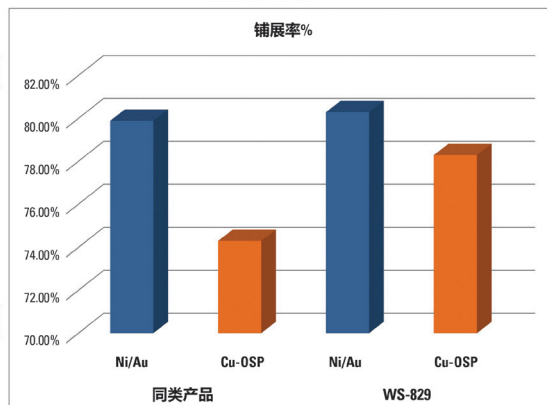
润湿性比较
