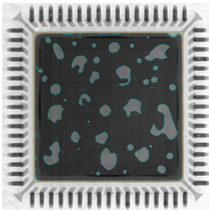
SAC305 T4
