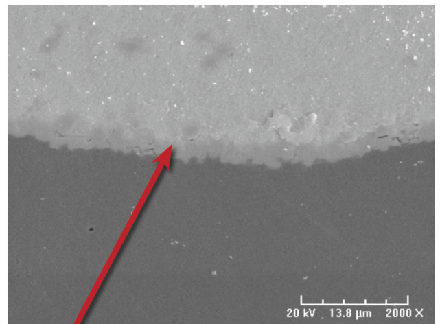
IMC Layer
